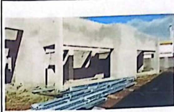
IMAGEM 08: Execução de reboco e emboço e material da estrutura da cobertura
